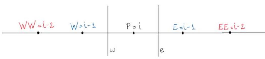
Fig. 118: Volume de controle com um nó central e dois nós à montante e à jusante
