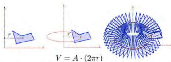
Fig. 156: Teorema de Pappus-Guldin - Autoria própria
