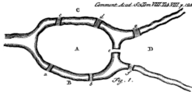
Fig. 183: Representação esquemática das pontes da cidade
