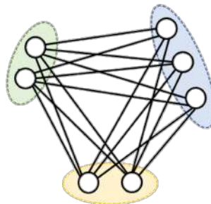
Fig. 184: Grafo tripartido completo K_{2,2,3} .
