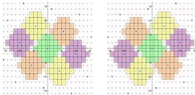
Fig. 199: Empacotamento dos reticulados \mathbb{L}_{a,25}\{(1, 7), (0, 25)\} e \mathbb{L}_{a,25}\{(1, 18), (0, 25)\} , respectivamente
