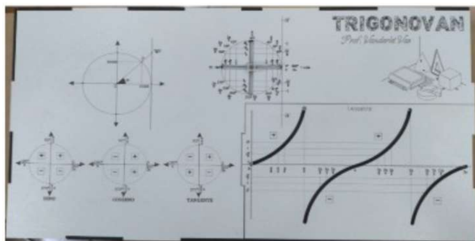
Fig. 83: Esboço da função tangente
