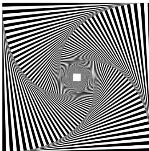
Fig. 95: Rotações e contrações de um quadrado
