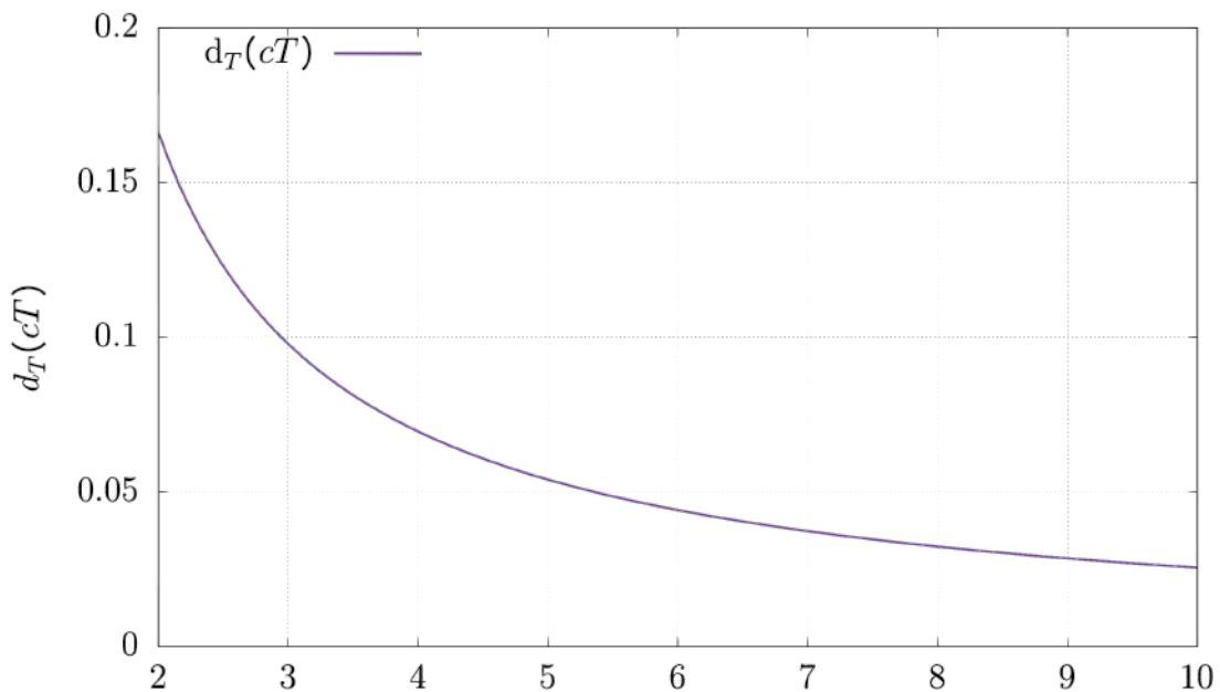
Fig. 182: Gráfico da função d_T(cT) definida pelo Teorema 9.44.
