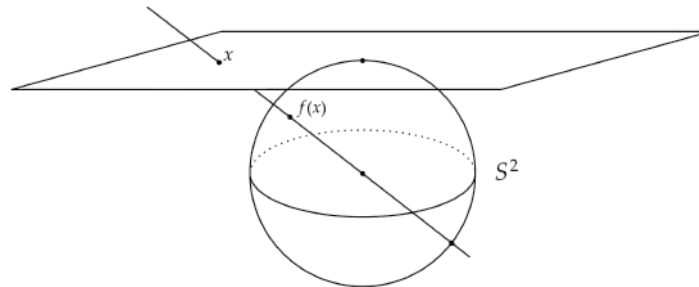
Fig. 167: Compactificação de \mathbb{R}^2 na esfera S^2 .
