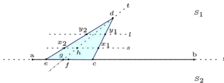
Fig. 125: Polígono de três lados.
