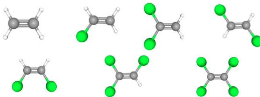
Fig. 110: Na primeira linha, da esquerda para a direita, representações do eteno, do cloroeteno, do 1,1-dicloroeteno e do trans-1,2-dicloroeteno. Na segunda, do cis-1,2-dicloroeteno, do tricloroeteno e do tetracloroeteno.
