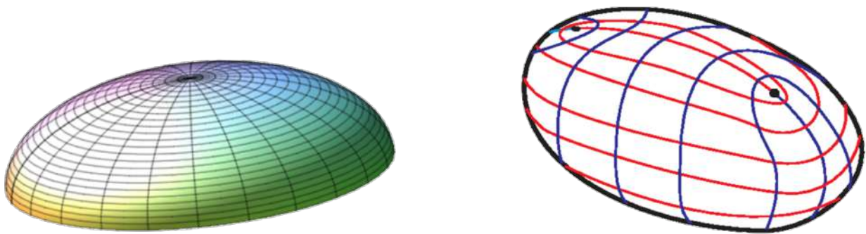
Fig. 87: Semi-elipsoide de revolução, à direita. Elipsoide de Monge, à esquerda.
