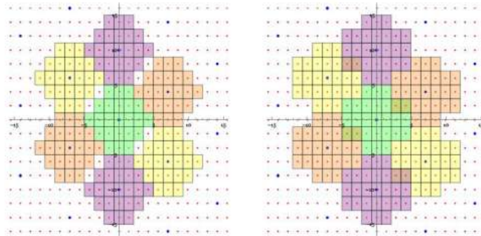
Fig. 198: Empacotamento e cobertura do \mathbb{L}_{a,25}\{(2, 5), (0, 5)\}
