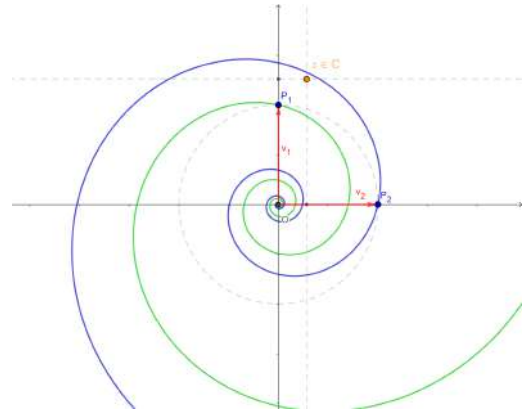
Fig. 21: Diagrama de fase de um sistema linear com autovalores complexos no caso em que \alpha, \beta > 0 .
