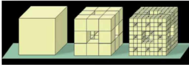
Fig. 179: Esponja de Menger
