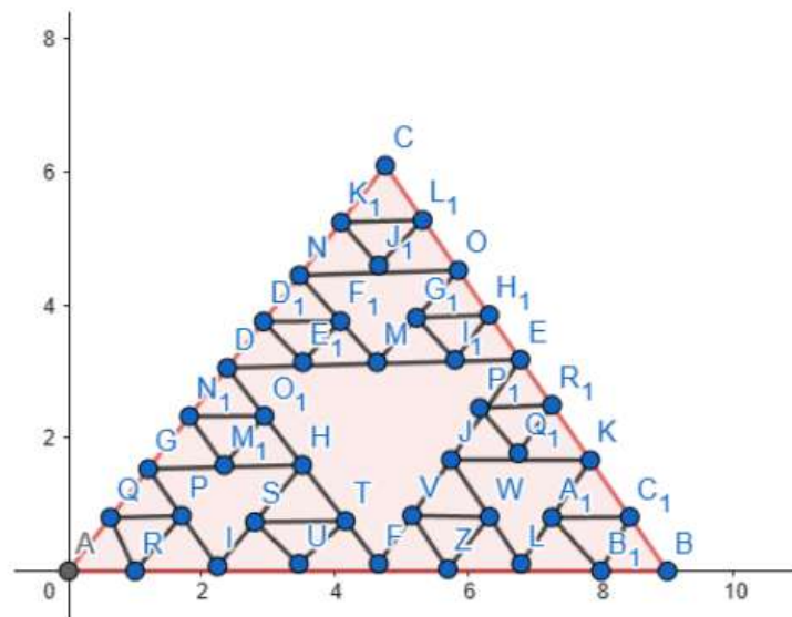
Fig. 5: O Triângulo de Sierpinski no Geogebra
