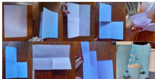
Fig. 119: Construção do Cartão Triângulo de Sierpinski
