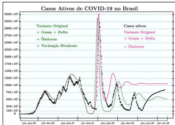
Fig. 53: Número de casos ativos de COVID-19 obtidos de [6] e o resultado da simulação usando o modelo SCEAIRD, com inclusão das variantes Gama, Delta e Ômicron e a vacinação com a Comirnaty ® Bivalente. Produzido pelos autores. Desenvolvido no software Wolfram Mathematica ® .
