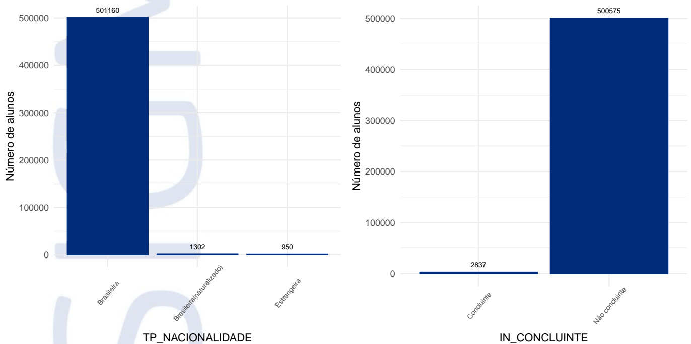
Figura 5: Frequência de alunos Ingressantes para as variáveis TP_NACIONALIDADE e IN_CONCLUINTE.
