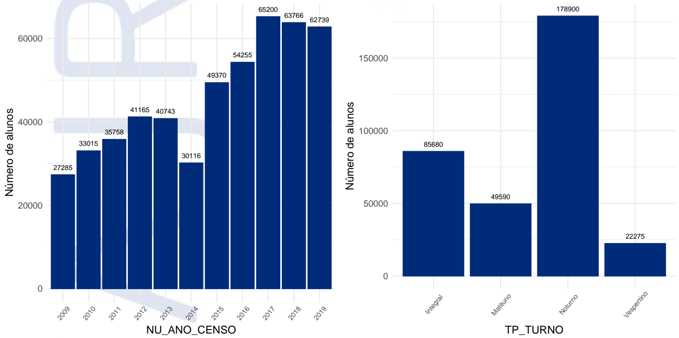
Figura 6: Frequência de alunos Ingressantes para as variáveis NU_ANO_CENSO e TP_TURNO.
