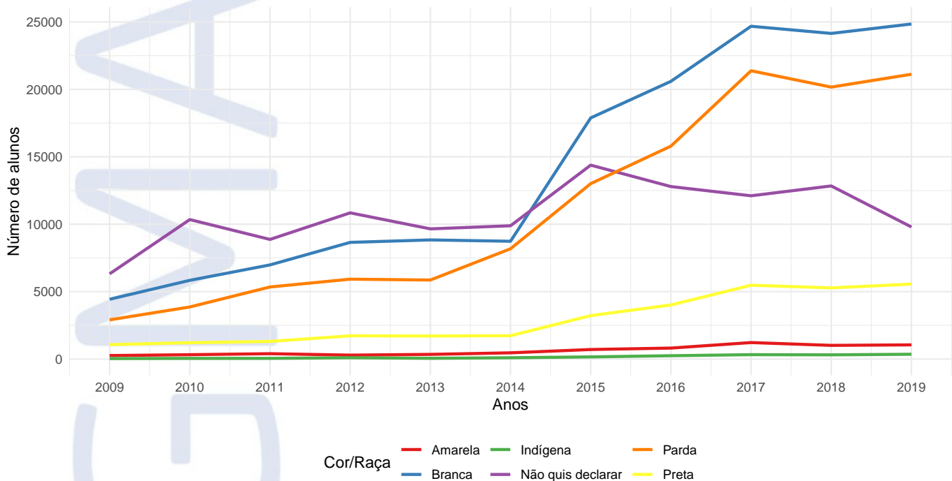
Figura 10: Frequência absoluta de alunos Ingressantes para a variável TP_COR_RACA entre os anos de 2009 a 2019.
