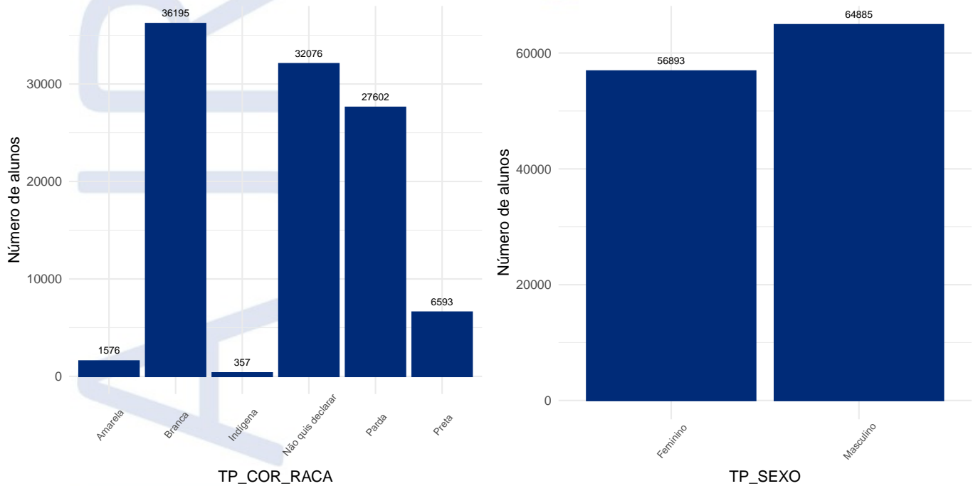
Figura 14: Frequência de alunos Formados para as variáveis TP_COR_RACA e TP_SEXO.
