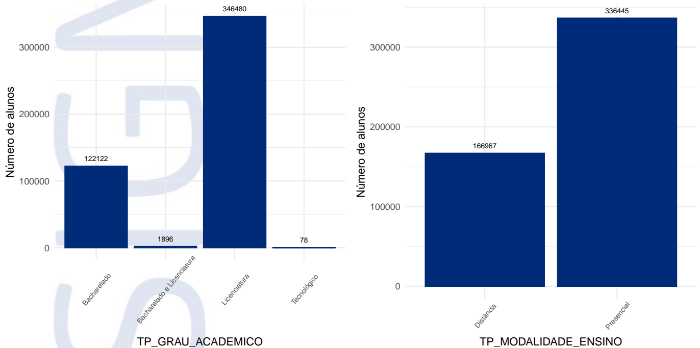
Figura 3: Frequência de alunos Ingressantes para as variáveis TP_GRAU_ACADEMICO e TP_MODALIDADE_ENSINO.
