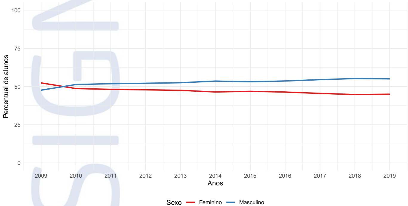
Figura 18: Frequência relativa de alunos Formados para a variável TP_SEXO entre os anos de 2009 a 2019.
