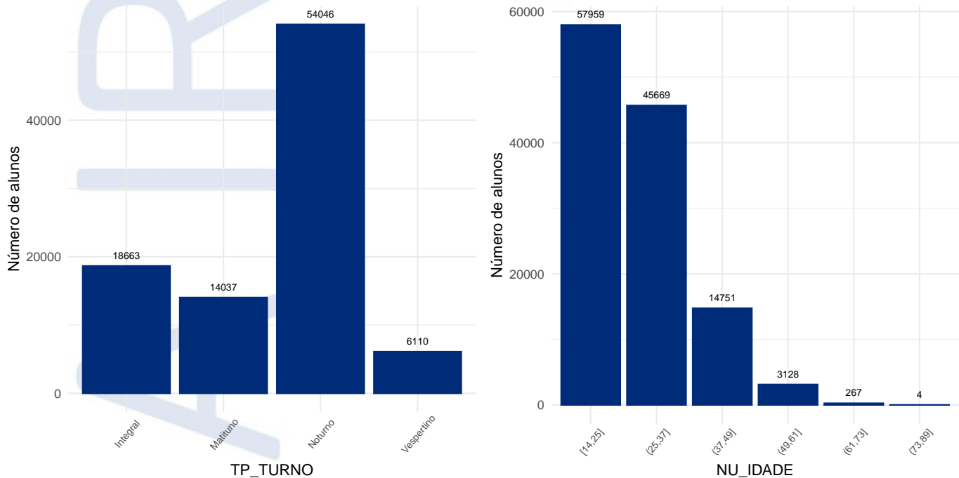
Figura 16: Frequência de alunos Formados para as variáveis TP_TURNO e NU_IDADE.
