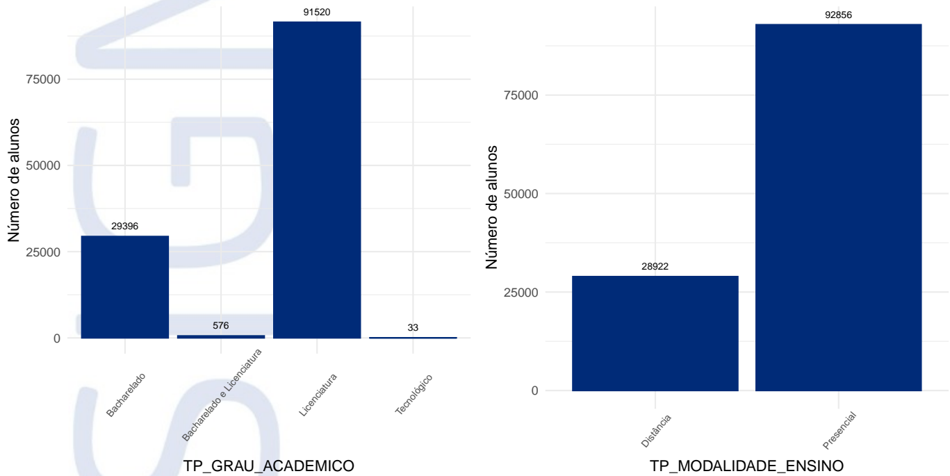
Figura 13: Frequência de alunos Formados para as variáveis TP_GRAU_ACADEMICO e TP_MODALIDADE_ENSINO.
